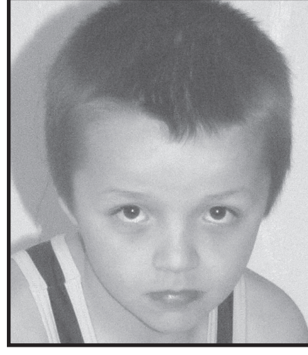
Dawson Holub
